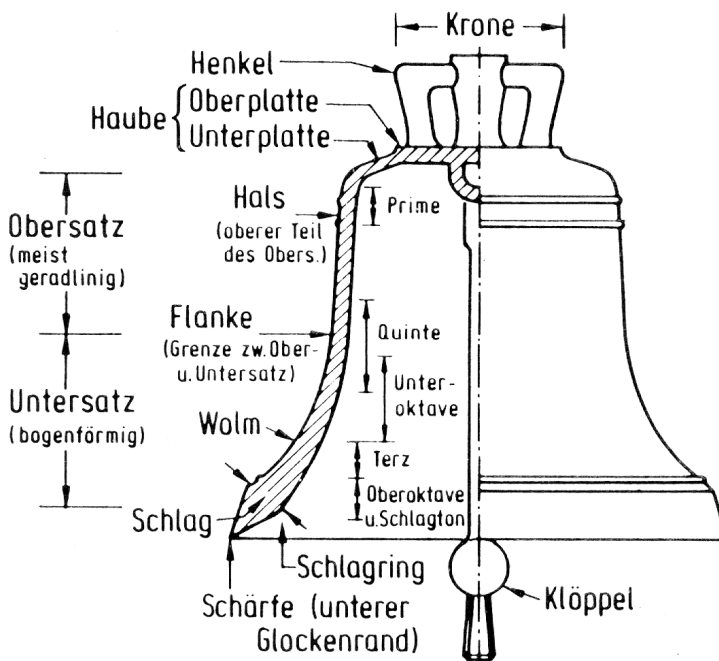
Abb.: 74 Zeichnung der Glocke teilweise im Schnitt Schnitt zur Begriffsbestimmung Glocke I
