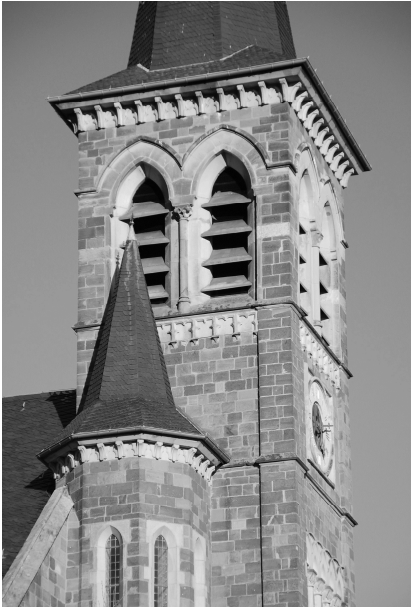
Abb. 130: Die Glockenstube vor der Umgestaltung mit den alten Klangjalousien. Deutlich zu erkennen ist der weite Abstand der Jalousien. Eine Klangverschmelzung konnte in diesem Zustand nicht erreicht werden.
